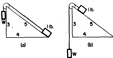
Fig. 4-3. Inclined plane.
