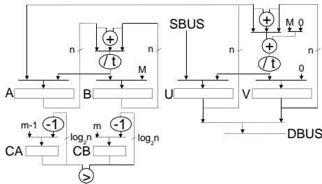
Fig. 8. Divider.
