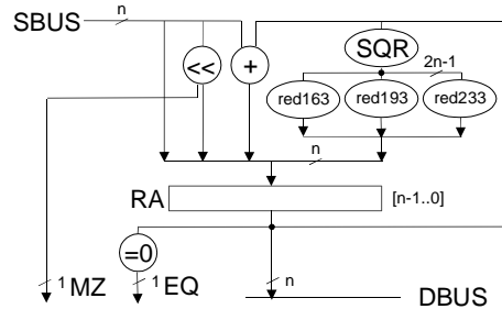
Fig. 5. ALU.
